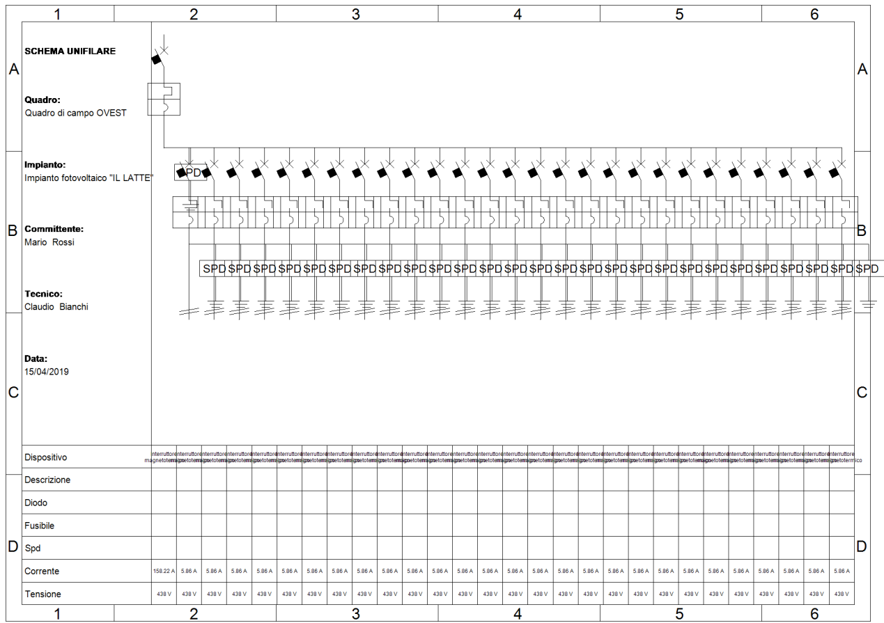
Fig. 6: Schema unifilare quadro "Quadro di campo OVEST"
