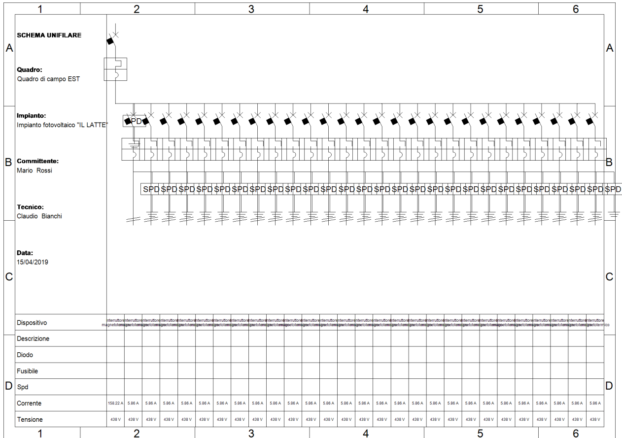
Fig. 7: Schema unifilare quadro "Quadro di campo EST"
